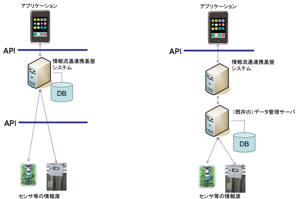
(a) 情報源・アプリケーションともに情報流通連携基盤の API に準拠
