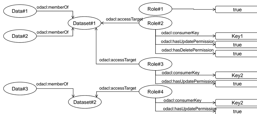
図 3.2: アクセス制御の記述例
