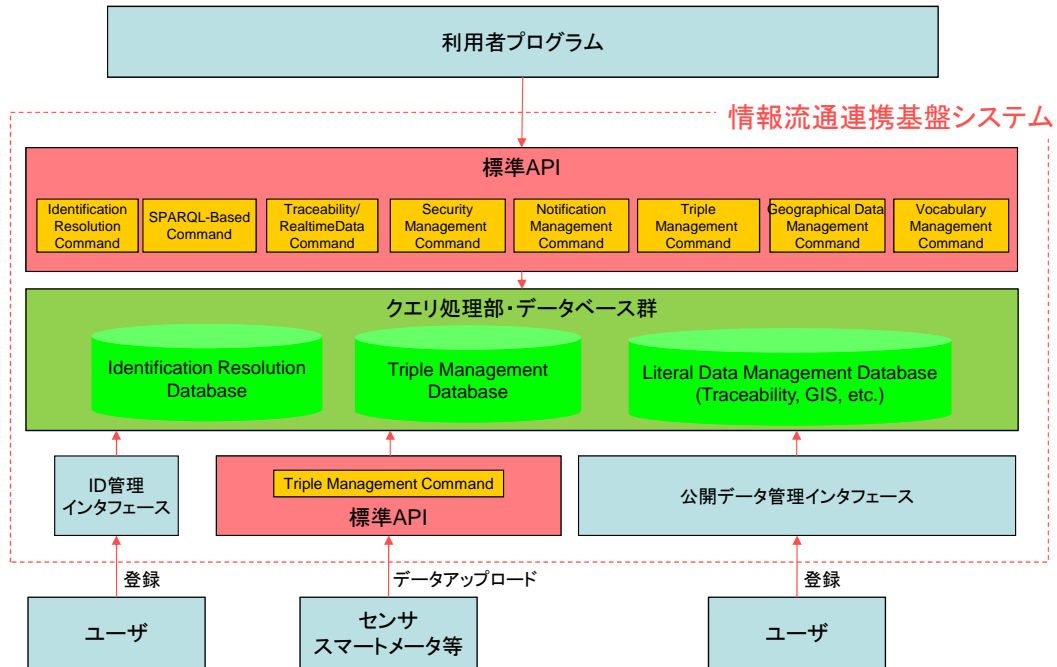
図 2.1: 情報流通連携基盤システムの構成
